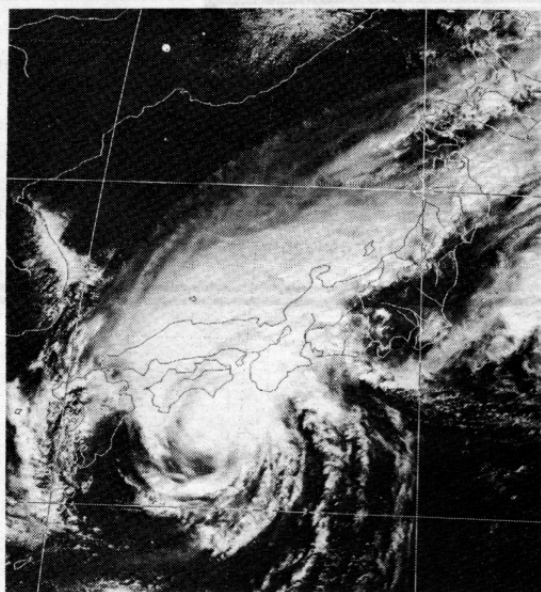
昭和55年10月14日、気象衛星「ひまわり」から送られてきた台風19号の写真
