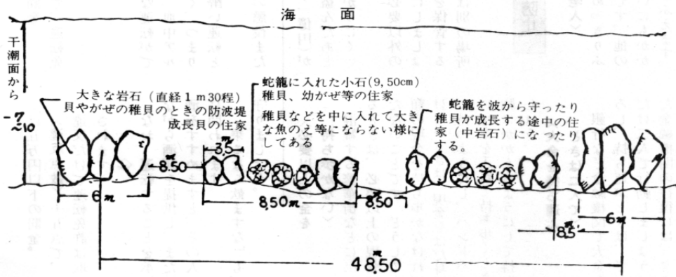
小川島稚貝保育場 断面見取図
